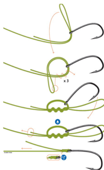
Goede variant op de palomarknoop
